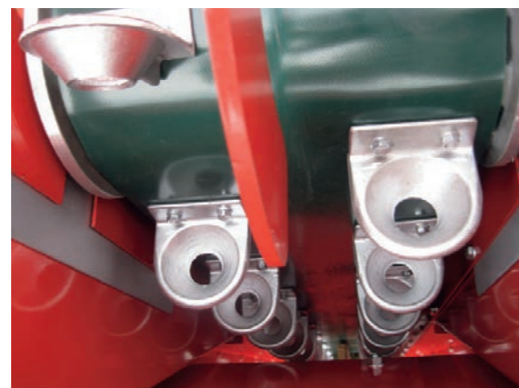
Tazzine per il carico del prodotto Buckets to load the product Godets pour le chargement du produit
